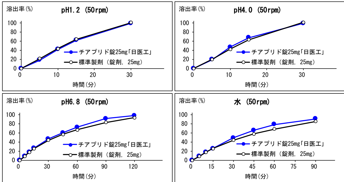
(溶出曲線)
