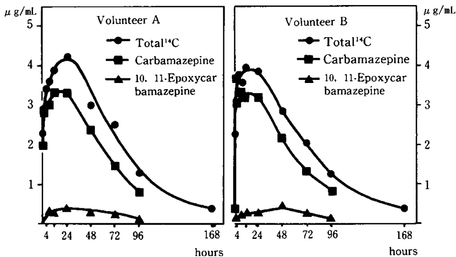
図 3 14 C-カルバマゼピン400mg経口投与後の血中濃度の推移
