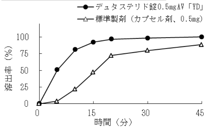
pH6.8 ホリソルベート 80 添加(0.5%(W/V)) (50回転)
