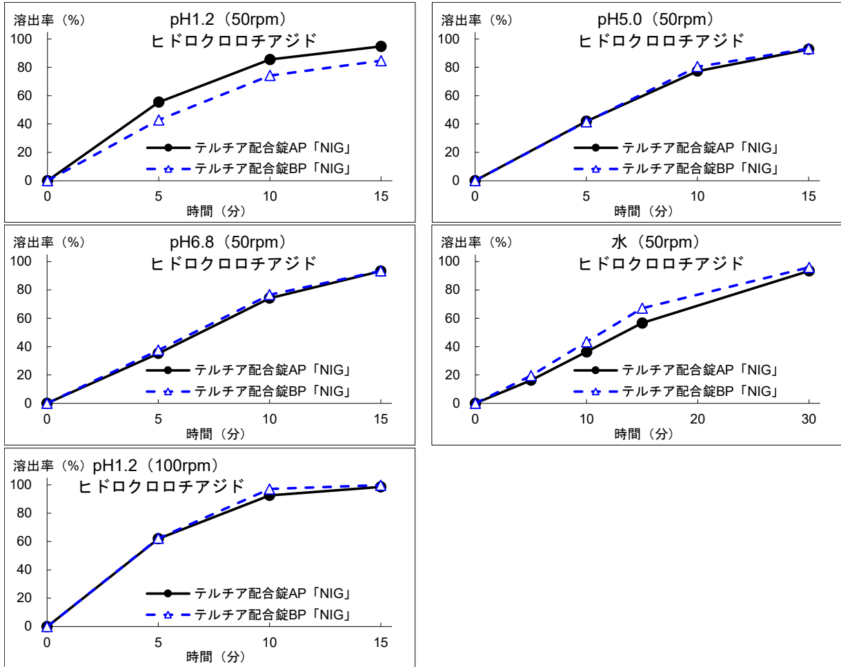
(溶出曲線)
