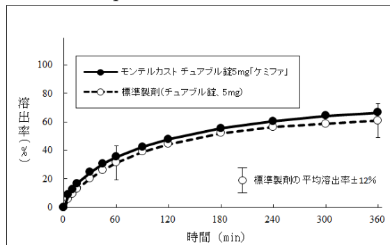
pH4.0 ポリソルベート 80 0.01%(W/V)添加 (50rpm) における溶出曲線
