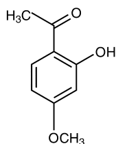
paeonol (ボタンピ)
