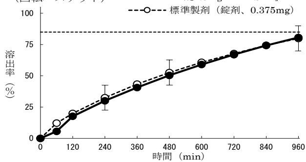
pH6.8/200rpm (回転バスケット)
