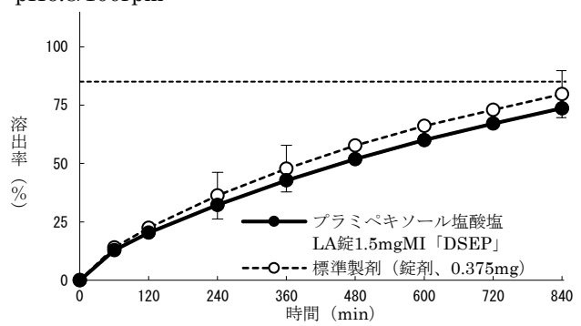
pH6.8/100rpm (回転バスケット)
