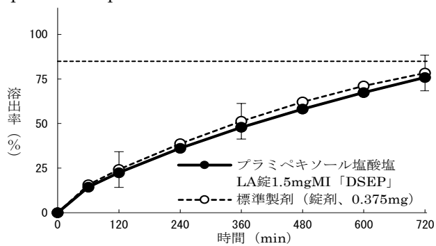
pH6.8/200rpm (回転バスケット)
