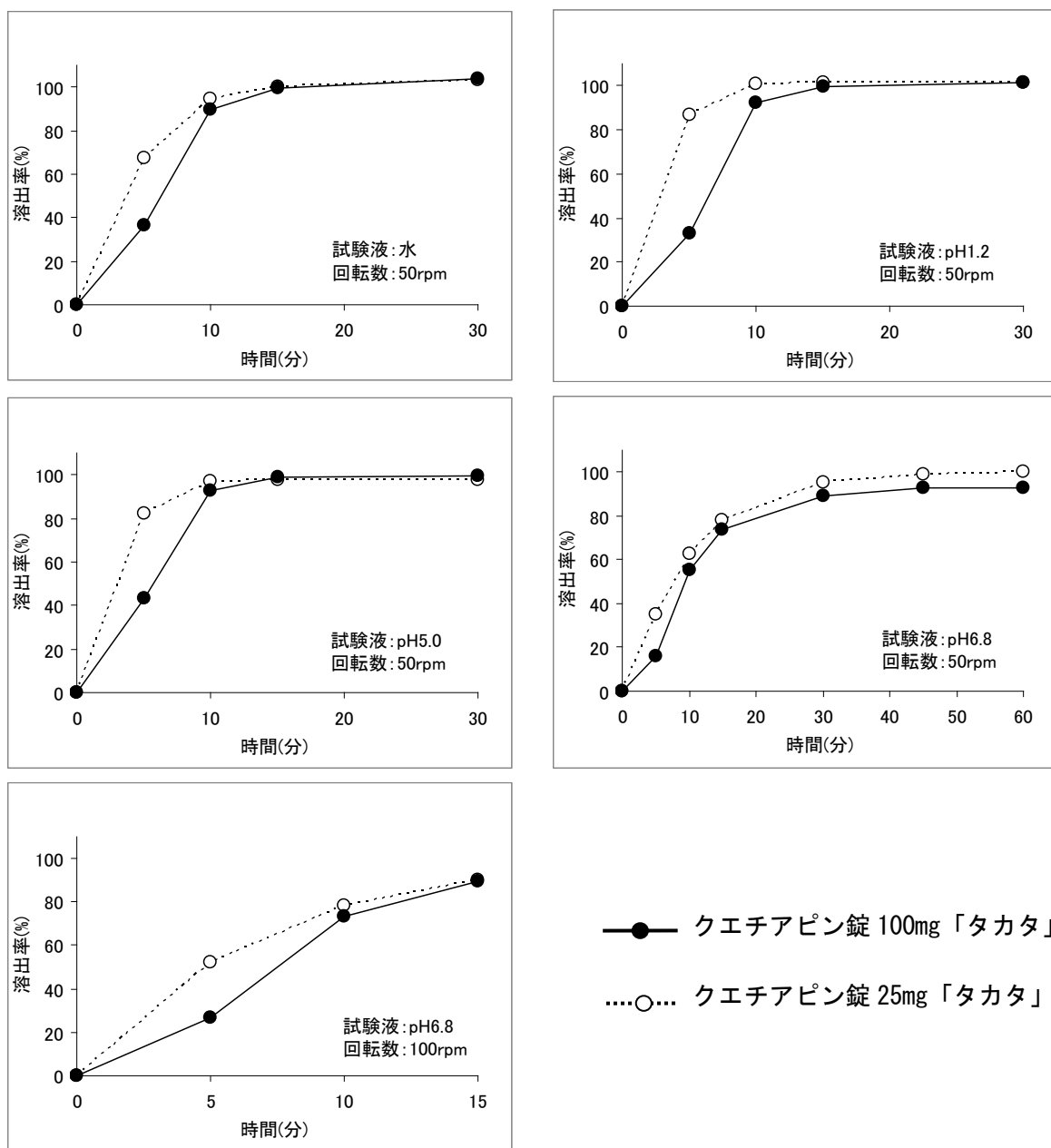
図 クエチアピン錠 100mg 「タカタ」とクエチアピン錠 25mg 「タカタ」の平均溶出曲線
