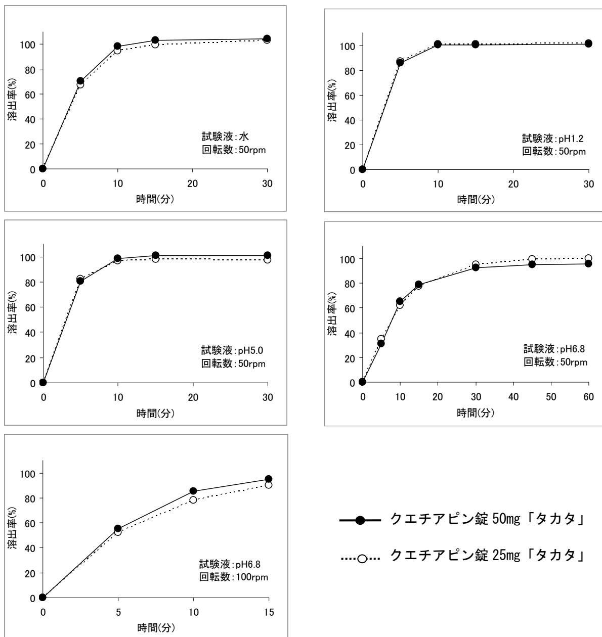
図 クエチアピン錠 50mg 「タカタ」とクエチアピン錠 25mg 「タカタ」の平均溶出曲線
