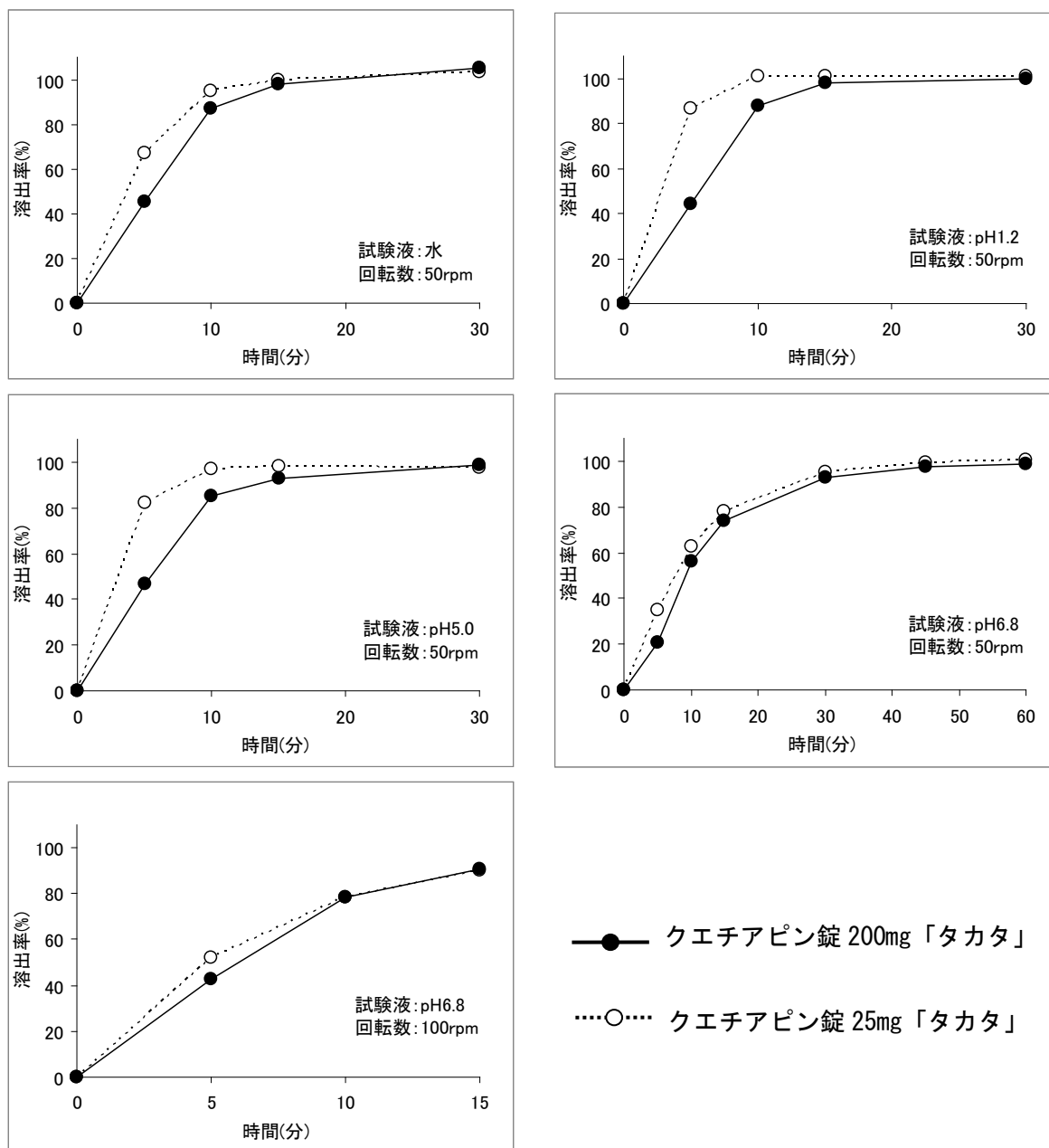
図 クエチアピン錠 200mg「タカタ」とクエチアピン錠 25mg「タカタ」の平均溶出曲線
