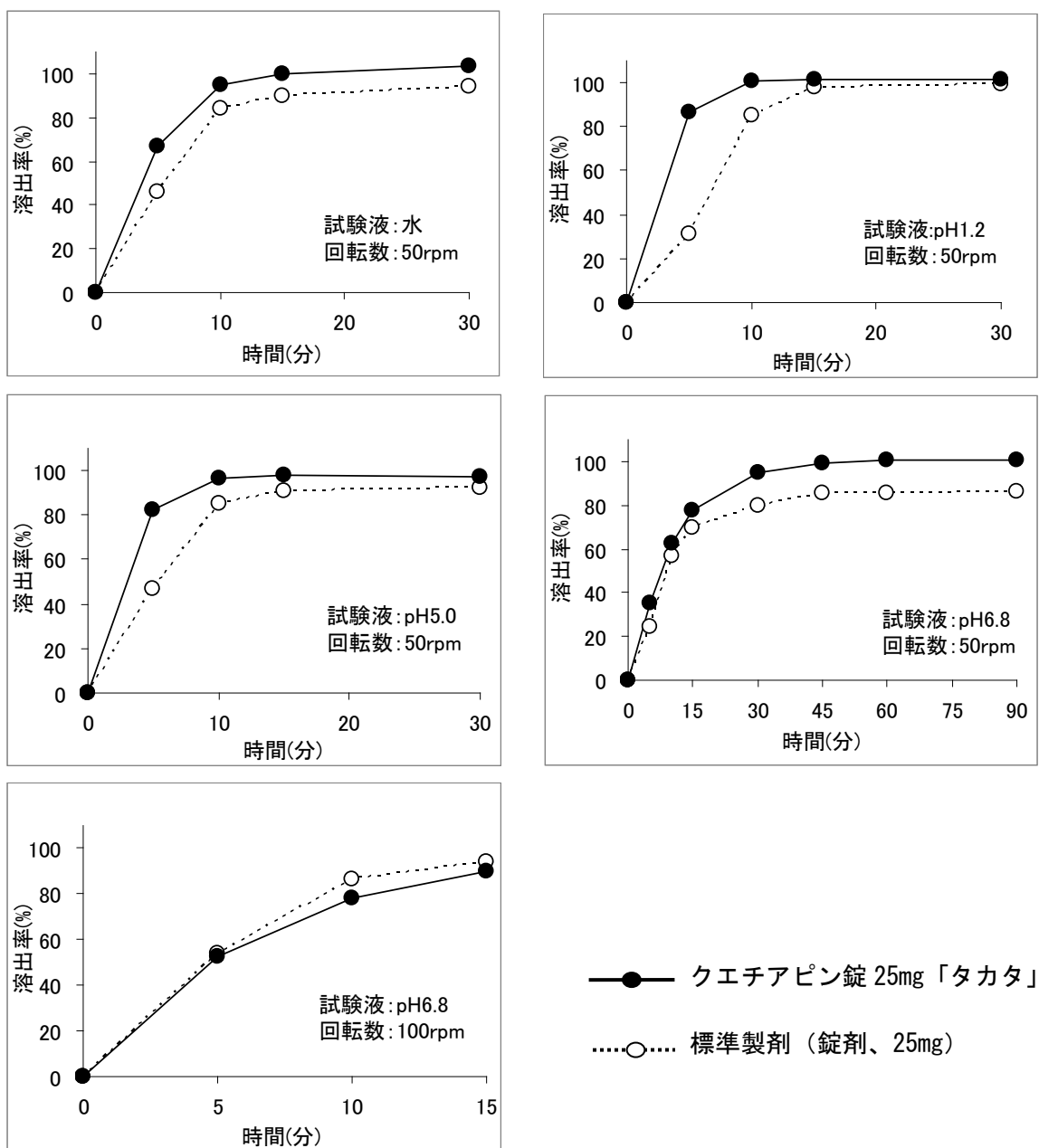
図 クエチアピン錠 25mg「タカタ」と標準製剤の平均溶出曲線
