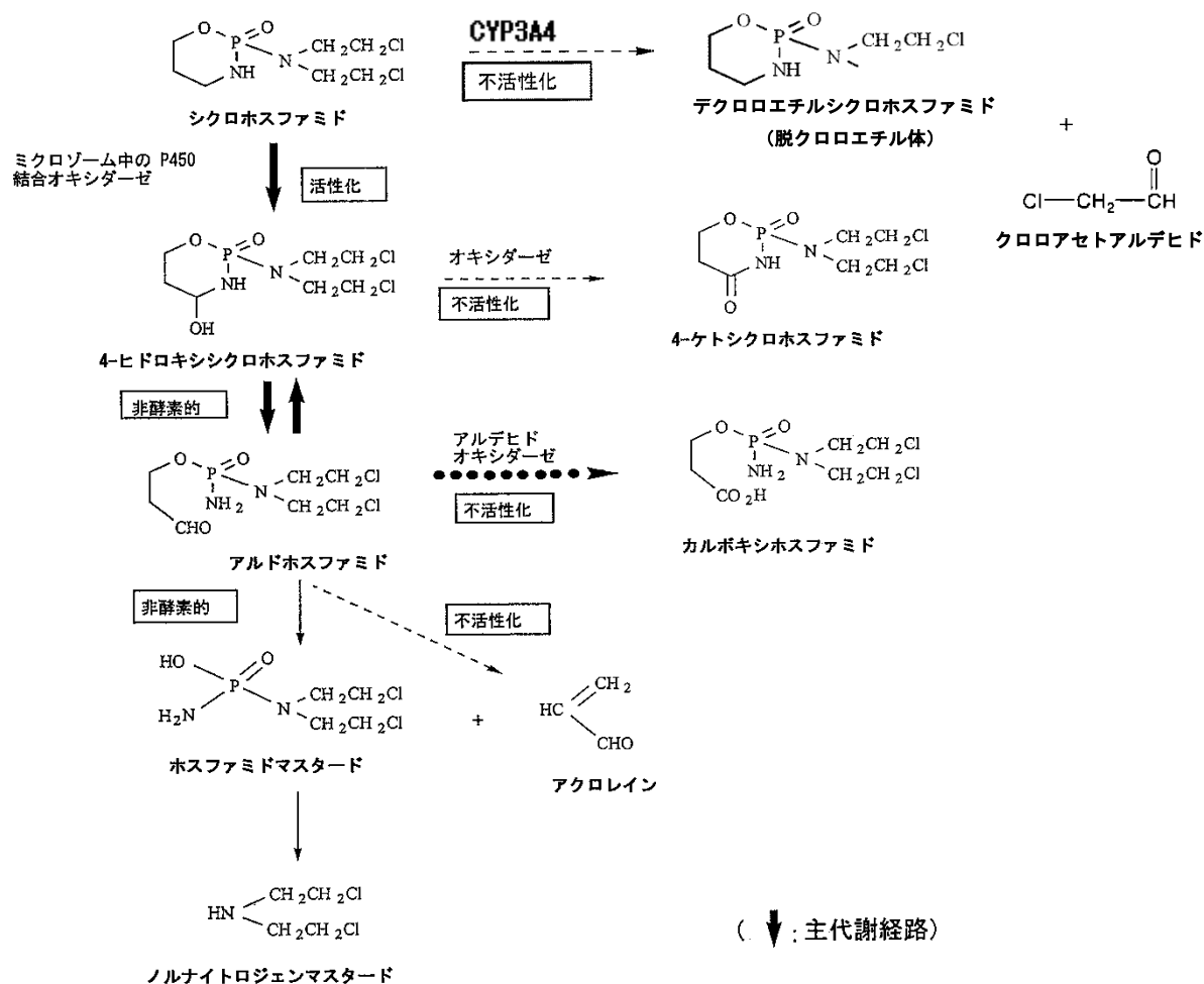
図VII-2 代謝経路
