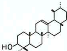
\alpha -amyrin
